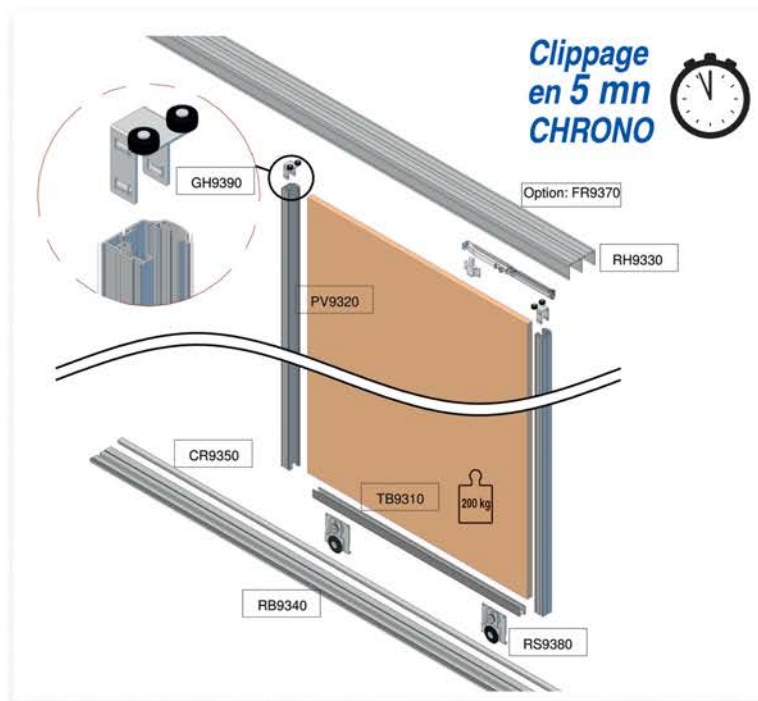
Panneau + traverse basse (Réf. TB9310)
