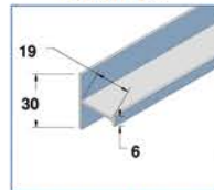
Traverse intermédiaire Réf. H1906
