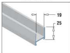
Traverse basse Réf. TB9310
